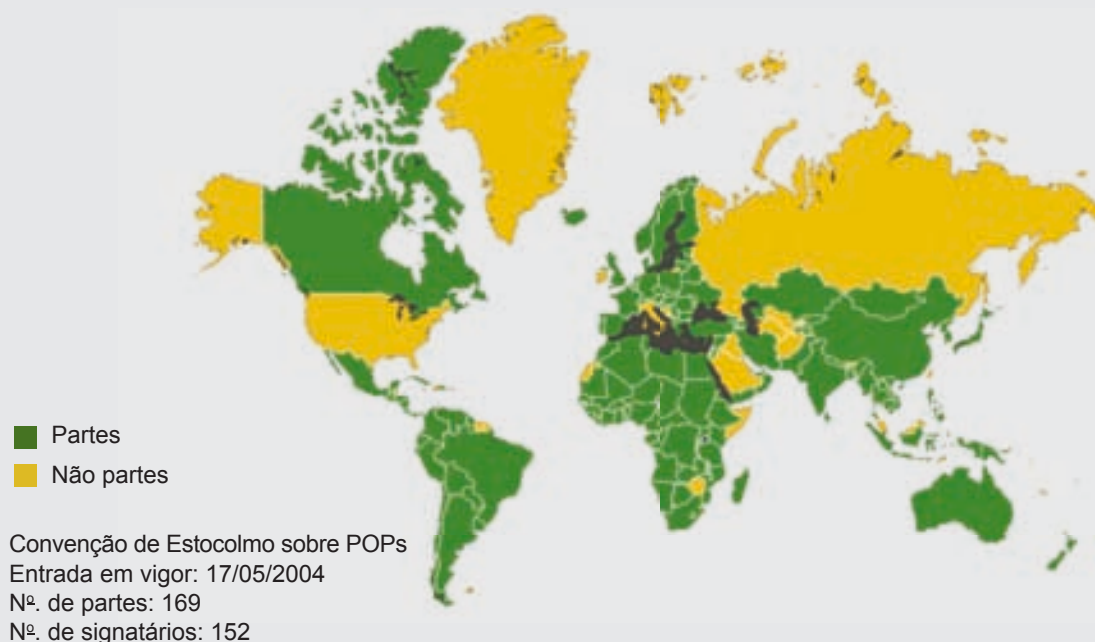
Figura 9. Situação da ratificação internacional da Convenção de Estocolmo sobre Poluentes Orgânicos Persistentes (partes da Convenção mostradas em verde)
