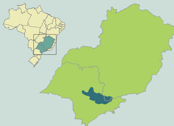
Figura 3. Localização das bacias dos Rios Piracicaba, Capivari e Jundiaí – Bacias PCJ
